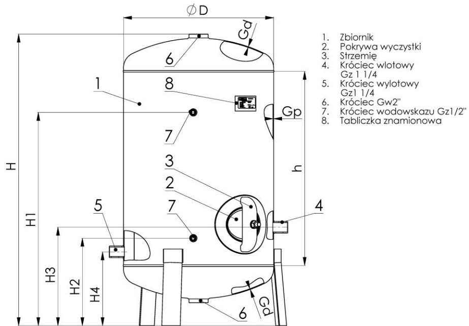
Rys.1 Zbiornik hydroforowy HVP151, HVP201, HVP301
