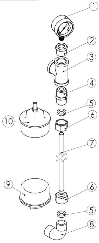
Rys. 4 Zestaw wyposażenia dodatkowego
