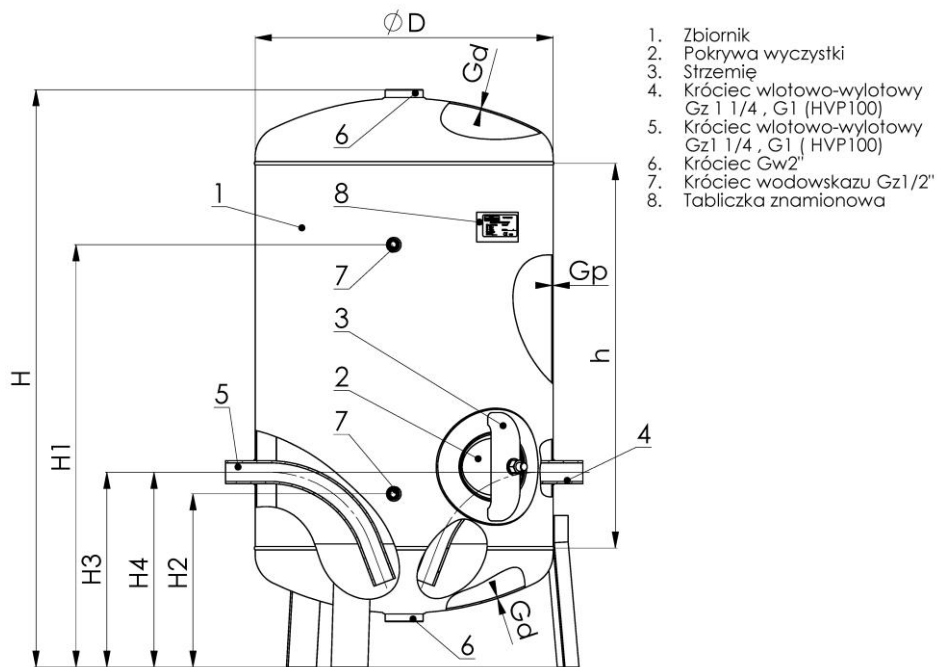
Rys.2 Zbiornik hydroforowy HVP100, HVP200, HVP300, HVP500
