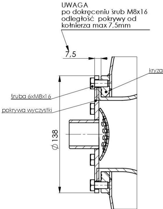
Rys.3 Montaż pokrywy wyczystki ZBOL100, ZBOL150
