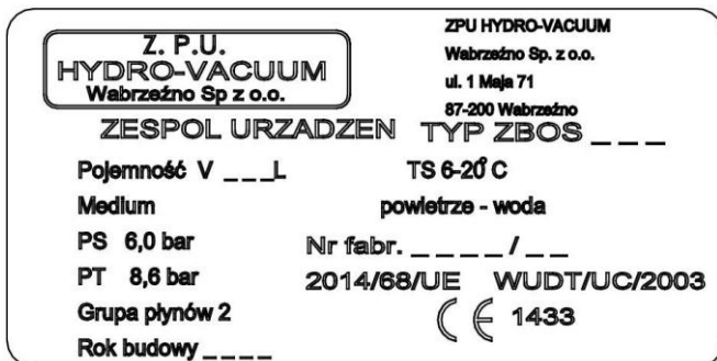
Rys. 1. Tabliczka znamionowa
