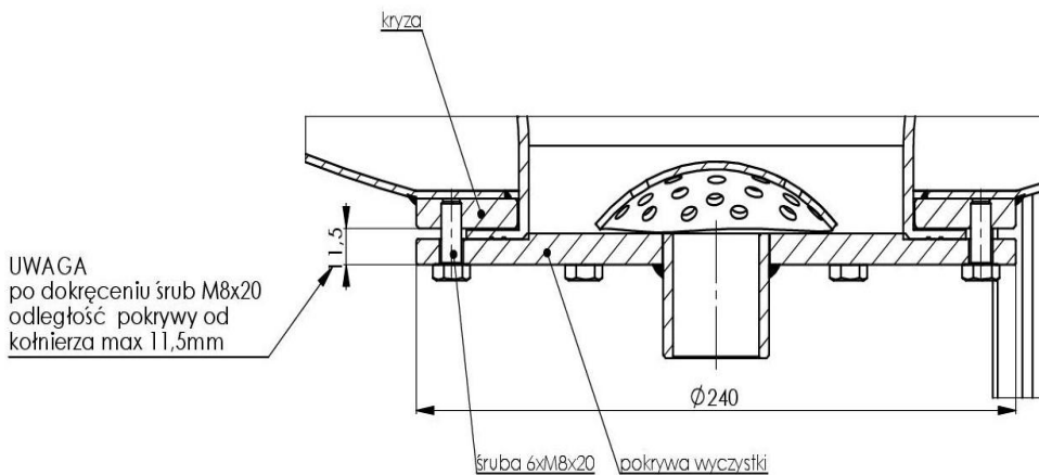
Rys.4 Montaż pokrywy wyczystki ZBOS200, ZBOS300, ZBOS500
