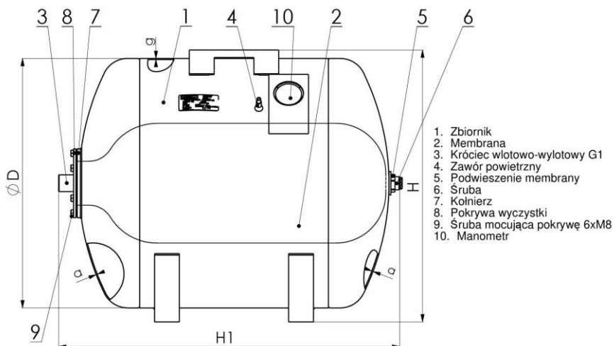
Rys.3 Dane techniczne zespołu urządzeń typ ZBOL100, ZBOL150, ZBOL200
